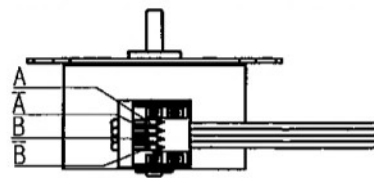
电机接线图
